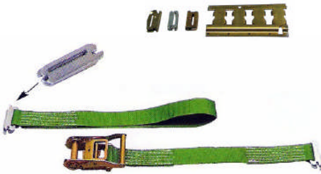
Sangle DR avec ridelles pour rail Sjorbanden met sleufgatenfitting nr 7
